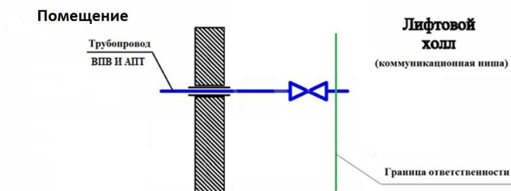
Схема присоединения помещения Владельца:
