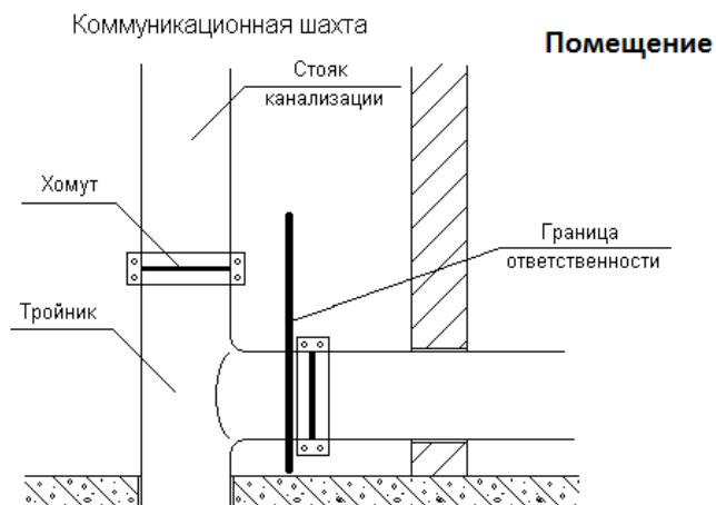
Схема присоединения Помещения Владельца:
