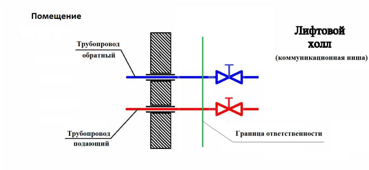
Схема присоединения Помещения Владельца:
